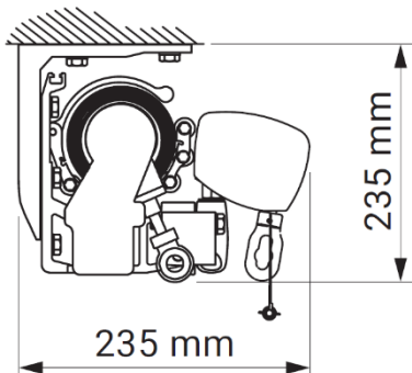
Montert i tak
