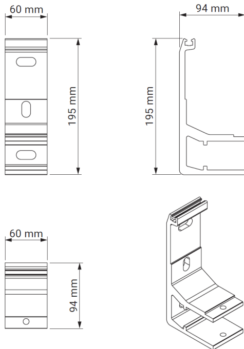
Veggbrakett
